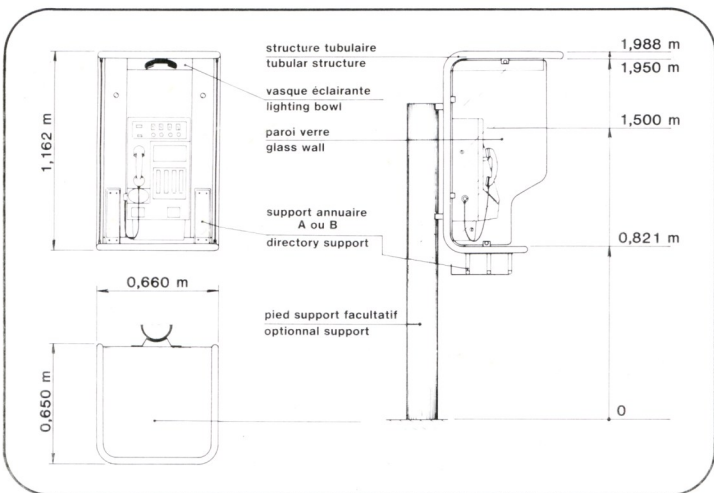
plan 3 vues
