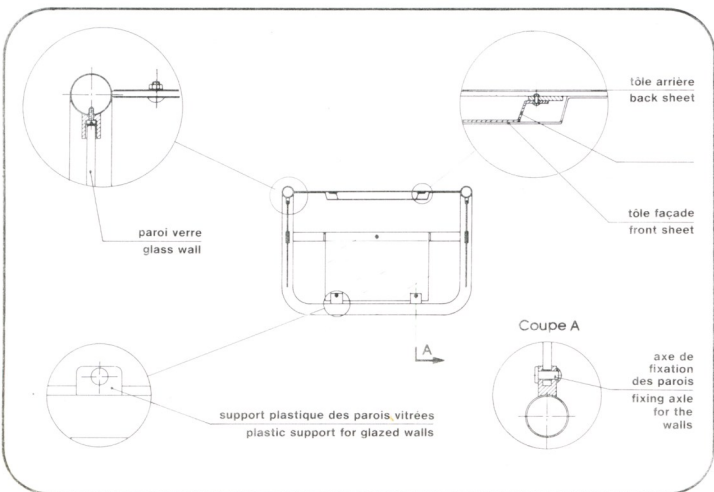
coupe horizontale
