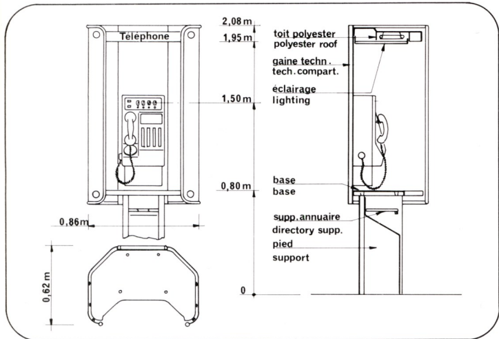
plan 3 vues
